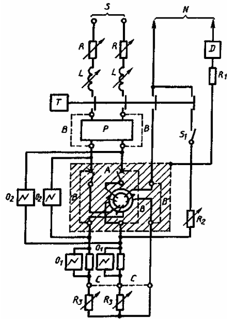
Рисунок 7 — Схема испытательной цепи для проверки правильности координации с аппаратом защиты от коротких замыканий и номинальной включающей и отключающей способности двухполюсного УЗО — Д с тремя путями прохождения тока без встроенной защиты от коротких замыканий в однофазной цепи со средней нейтралью
