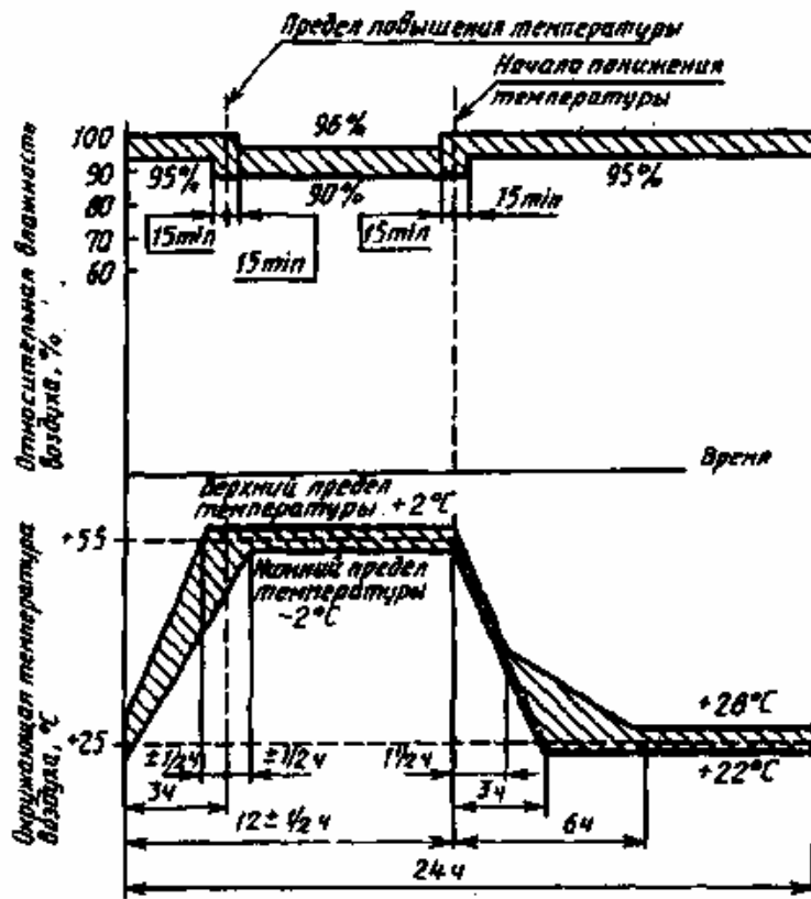
Рисунок 12 — Цикл испытания
