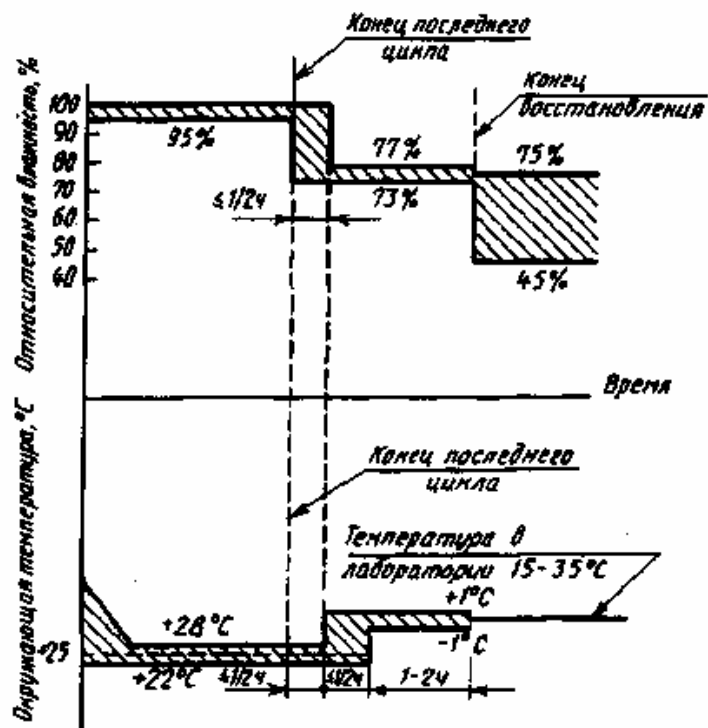
Рисунок 13 — Восстановление
