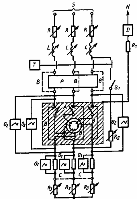
Рисунок 8 — Схема испытательной цепи для проверки правильности координации с аппаратом защиты от коротких замыканий и номинальной включающей и отключающей способности трехполюсного УЗО — Д без встроенной защиты от коротких замыканий в трехфазной цепи
