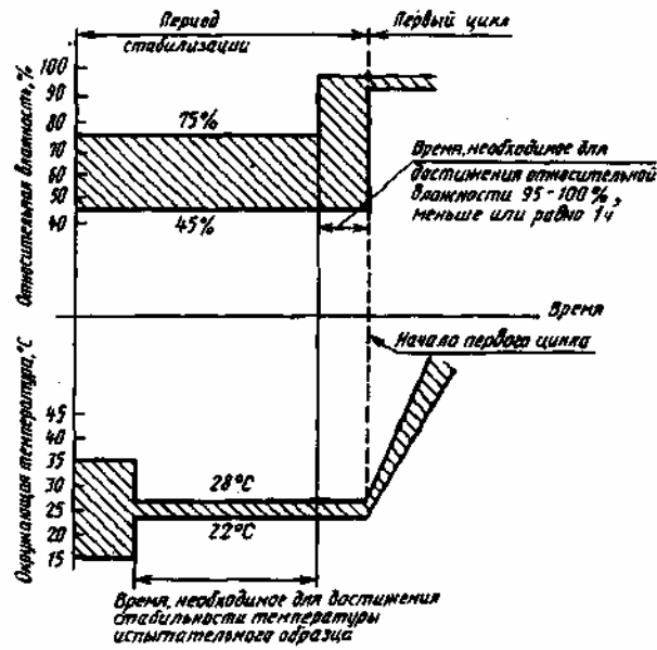
Рисунок 11 — Период стабилизации
